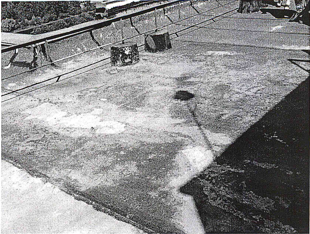
местами поврежден рулонный ковер кровли
